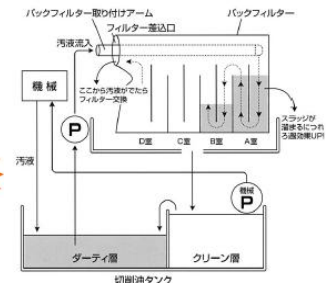
■切削油・クーラントろ過装置 EJV-40
